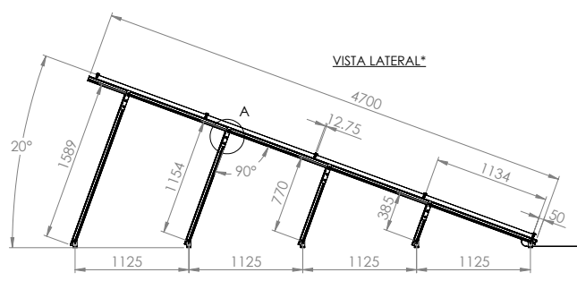
Modelo de 4 soportes.
